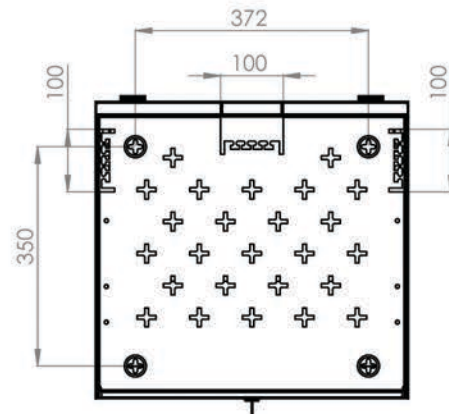
Vue arriere
