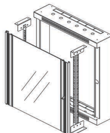
Système de verrouillage à 3 points
